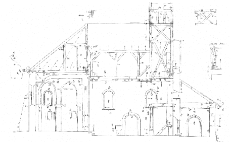
Jezero, crkva sv. Jurja, uzdužni presjek, terenski crtež, Davorin Stepinac, 1973.
