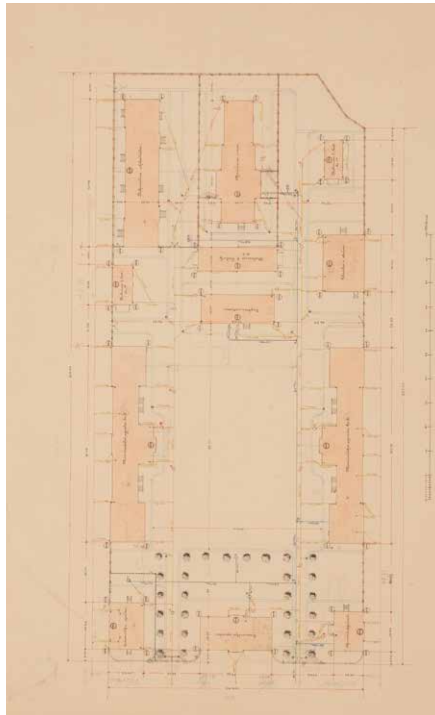
Domobranska vojarna, 1898., položajni nacrt (dvije varijante), DAZG
