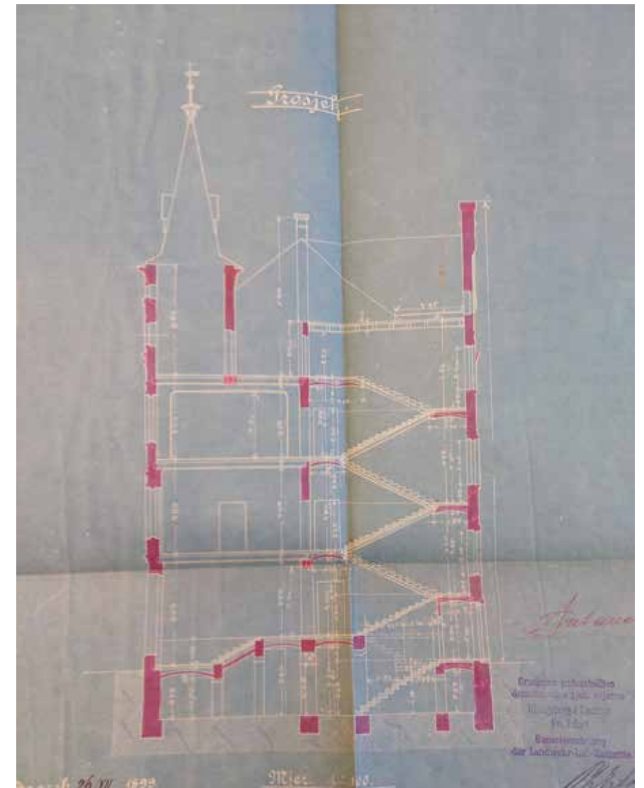
Presjek kroz stubište, izvedbeni projekt, 1899., DAZG
