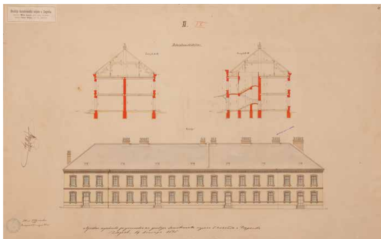
»Doknadna skladišta« (br. XI), projekt, 1898., DAZG
