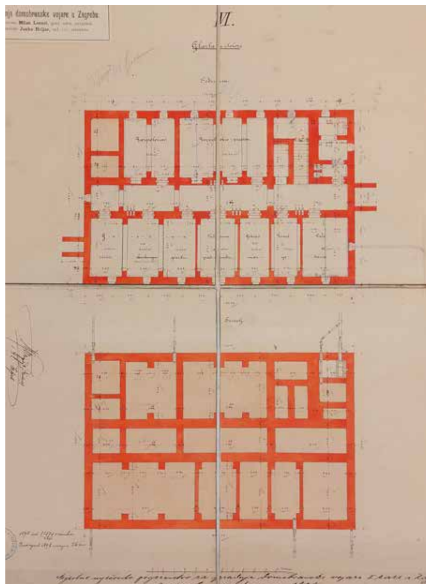
Zgrada za »glazbu i stožer« (br. VI), projekt, 1898., DAZG
