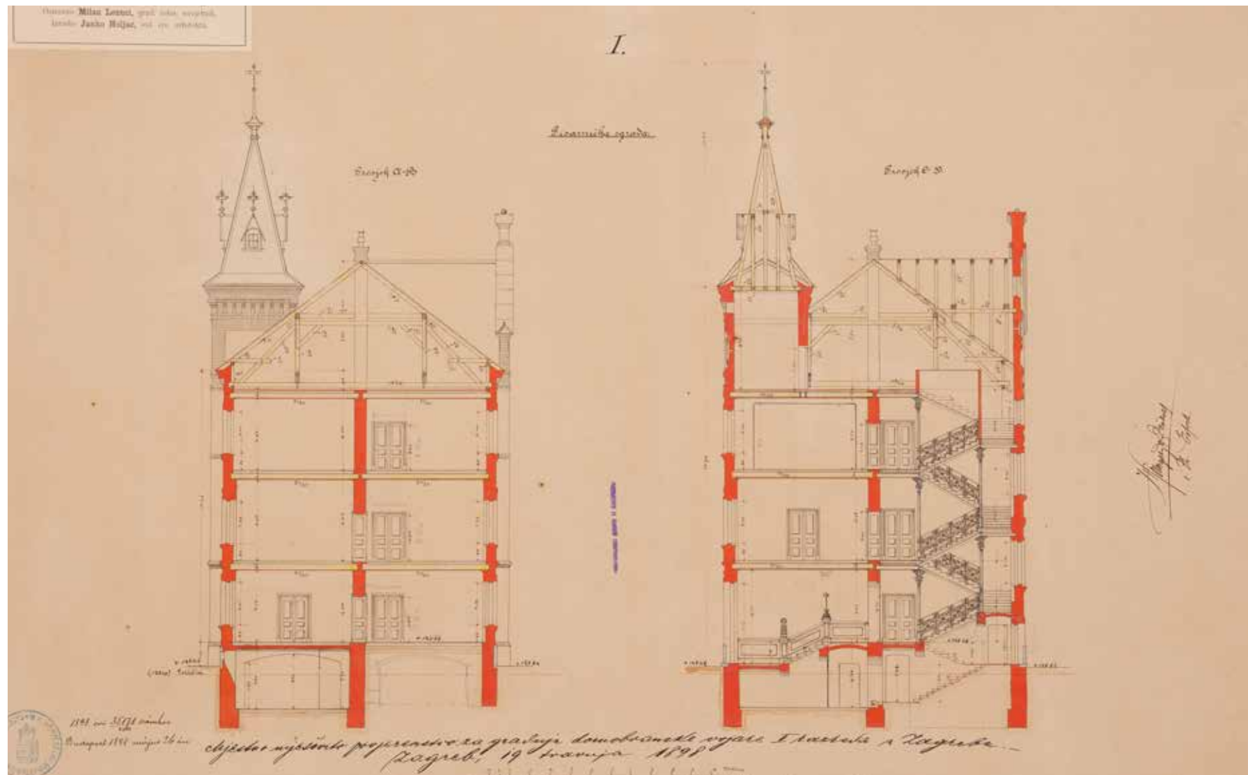
Presjek kroz bočne prostorije i kroz stubište, projekt, 1898., DAZG
