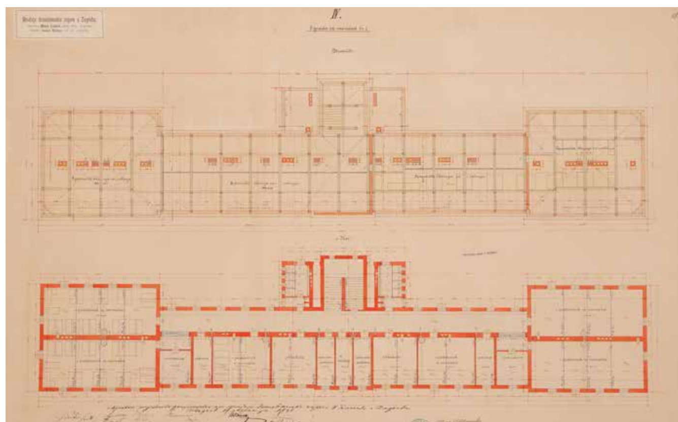
Momčadska zgrada (br. IV), projekt, 1898., DAZG
