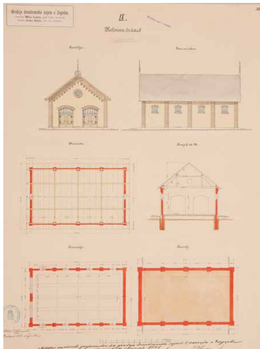
Kolnice (br. IX, X), projekt, 1898., DAZG
