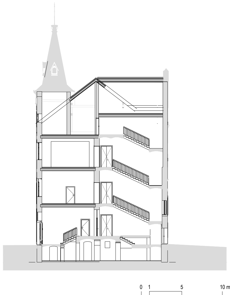
Poprečni presjek kroz stubište
