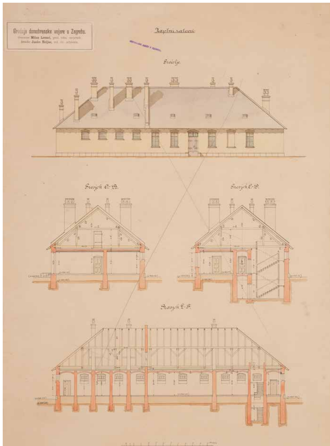
»Zaptni zatvor« (br. VII), projekt, 1898., DAZG
