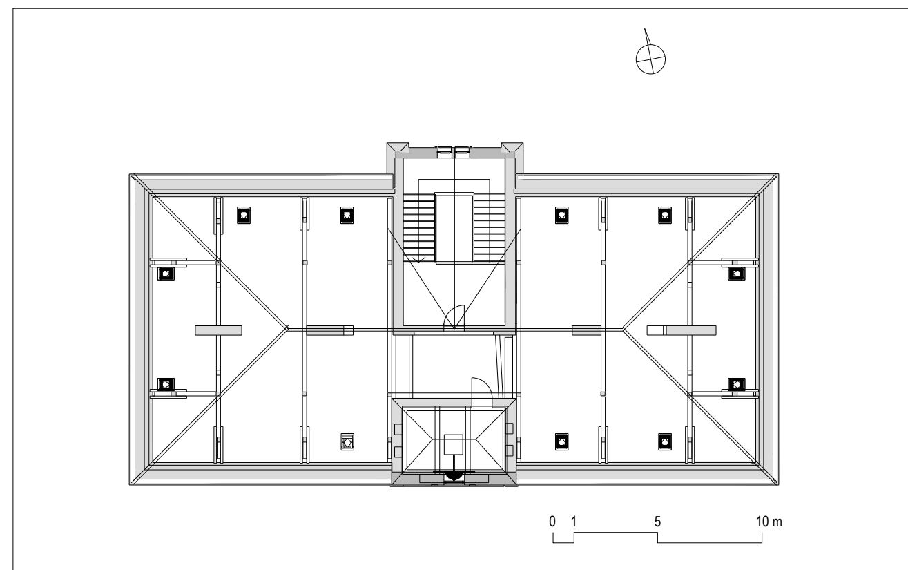
Tlocrt drugog kata i potkrovlja
