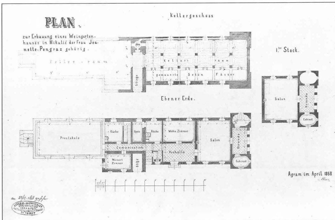
Tloort podruma, prizemlja i prvoga kata
