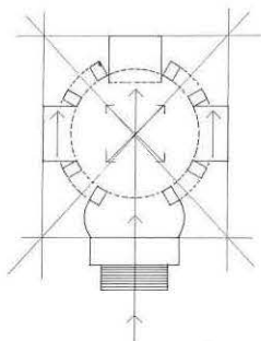
KARL VON KELLER Župna crkva, 1903.
