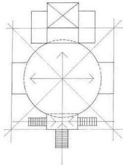
OTTO WAGNER Crkva u Währingu Beč, 1898.
