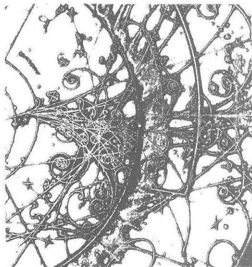
Putanje čestica
