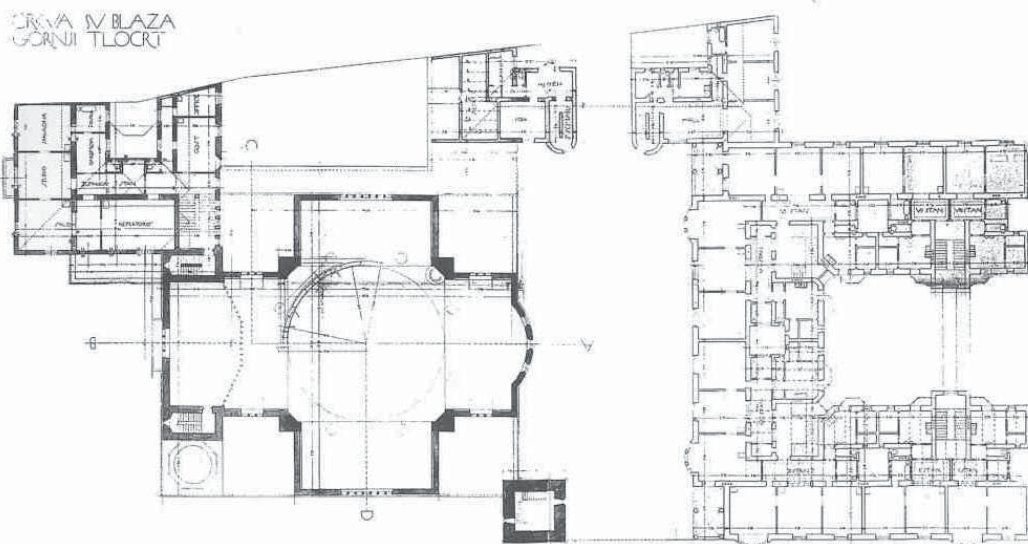
6 Viktor Kovačić, tlocrt pjevališta i prvog kata najamne stambene zgrade u Primorskoj ulici, listopad 1909. g./24.08.1910. g.
